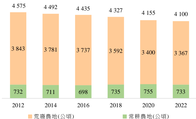
圖2 — 農地總面積
